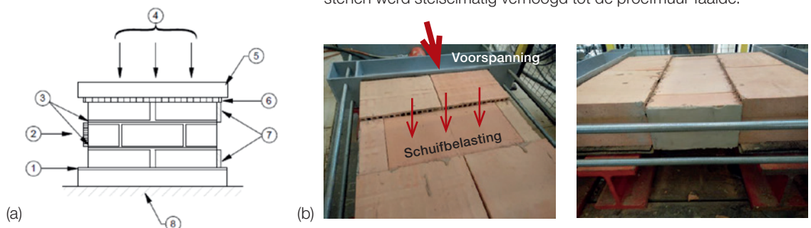
Figuur 1 (a) Testopstelling uit EN 1502-4. Deze zorgde voor falen door breuk van de middelste steen
