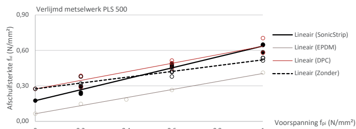
Figuur 2 Resultaat afschuifproeven SonicStrip, EPDM en DPC in verlijmd metselwerk PLS 500 (De Cooman & Deforce, 2018)
